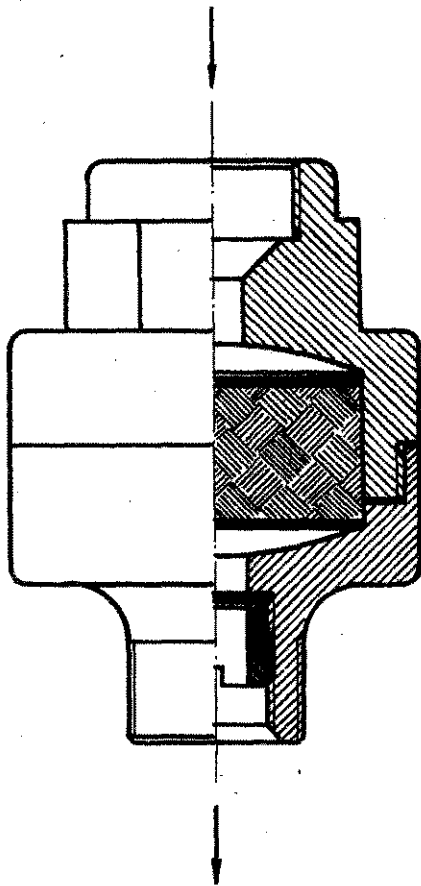
Drótbetétes lángvisszavágást gátló patron
