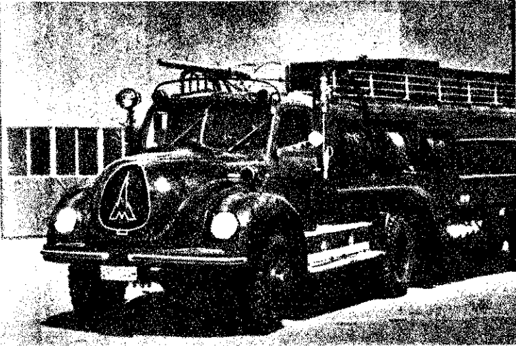
8000 liter vizet, 800 liter habképzőanyagot és kb. 1000 kg szén-savat szállít a Magirus-Deutz cég Uruguay részére készített tartályos gépjárműfűcsődjéje.
