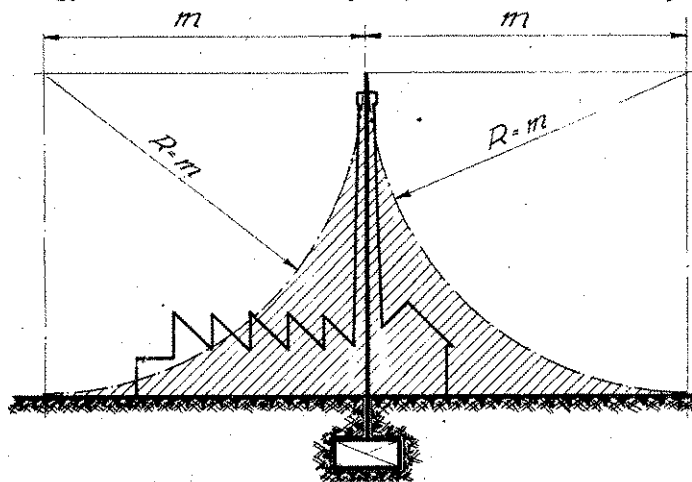
A gyárkémény villámhárítója részben a környezetet is veszélyeztet
