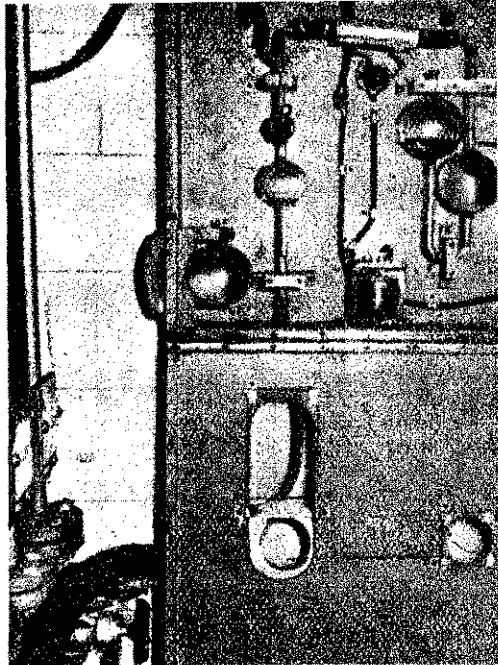
A hidrogéngáz szennyeződését kimutató készülék
