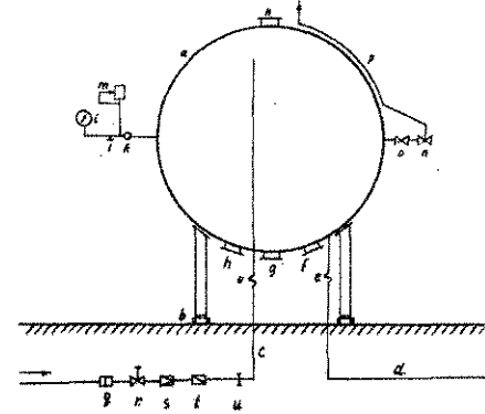
A gömbtartály metszete:
