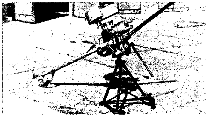
A búvárszivattyú motorjából készített csónakmotor
