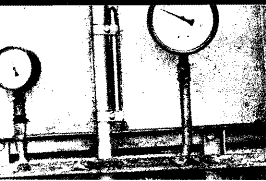
A gáz nyomását és mennyiségét műszerek segítségével ellenőrzik
