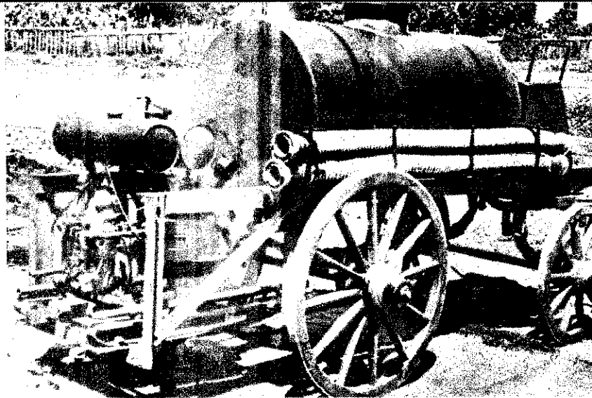
Íme az „összeházassított” lajtífecskeendő
