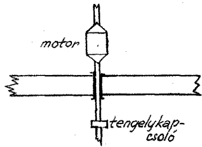
Az erőátvitel szigetelése a válaszfalon
