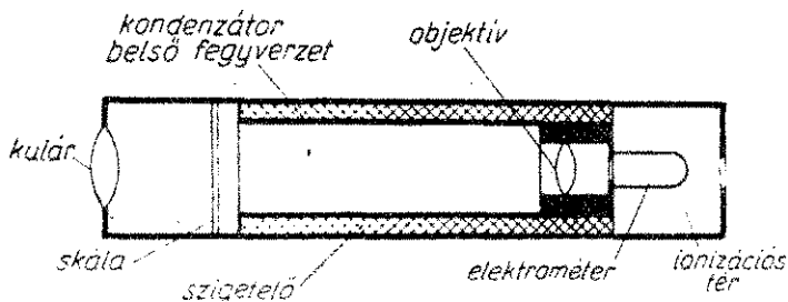
Közepes méréshatárú önleolvasó zsebdozismérő
