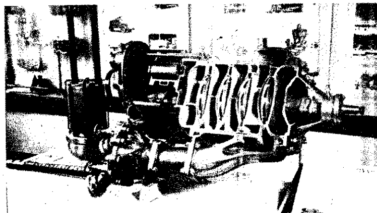
Niagara-szivattyú metszete
