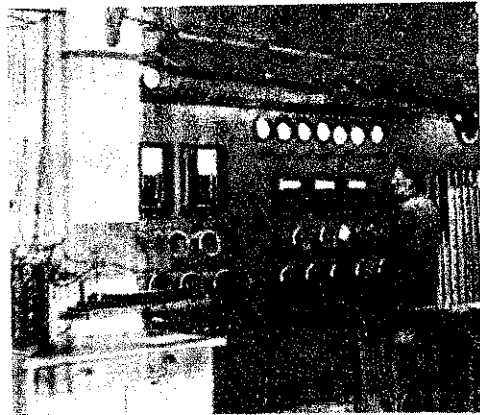
Műszertábla gázok megenged- hető nyomásának, hőmérsékle- tének és mennyiségének ellen- őrzésére
