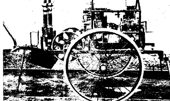
A targoncáról leemelhető 400 l/p-es kismotorfecskendő
