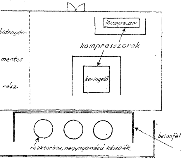
Az üzem elrendezése
