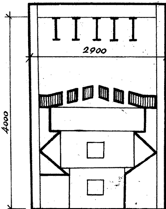
Gerenda és lépcsőfok vizsgálatára szolgáló kemence
