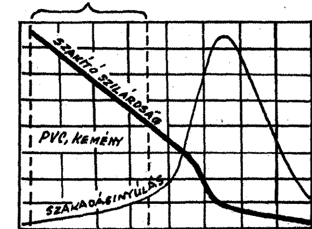
mény PVC szilárdsági értékeinek függése a hőmérséklettől
