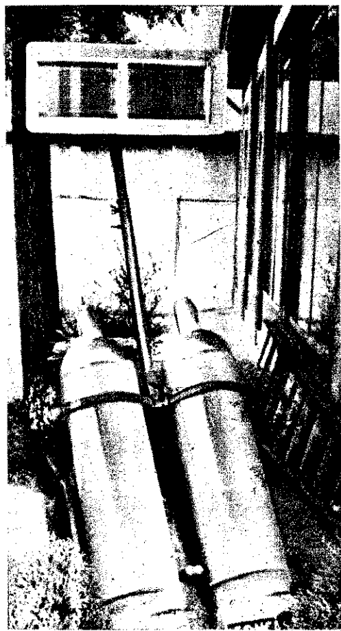
Propán-bután gázzal működő, targoncára szerelt hőszugárzó — üzemi célra
