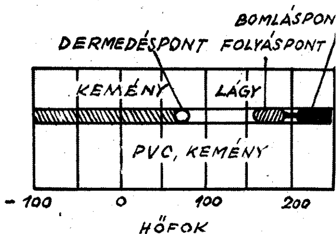
A PVC halmazállapotának függése a hőmérséklettől
