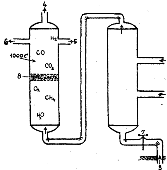
A hidrogén metánból történő előállításának vázlatos rajza. 1. Vízgőz — 2. Oxigén — 3. Metán fővezeték — 4. Vízgőz tisztító állomás — 5. Széndioxid — 6. Szénmonoxid — 7. Főelzáró csap. — 8. Nikkelvegyület-katalizátor
