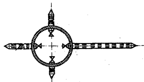
Csápos kút
