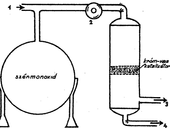
szénmonoxid további felhasználásának vázlata: 1. vízgőz bevezetése — 2. Nyomásfokozó szivattyú — 3. Hidrogén — 4. Széndioxid
