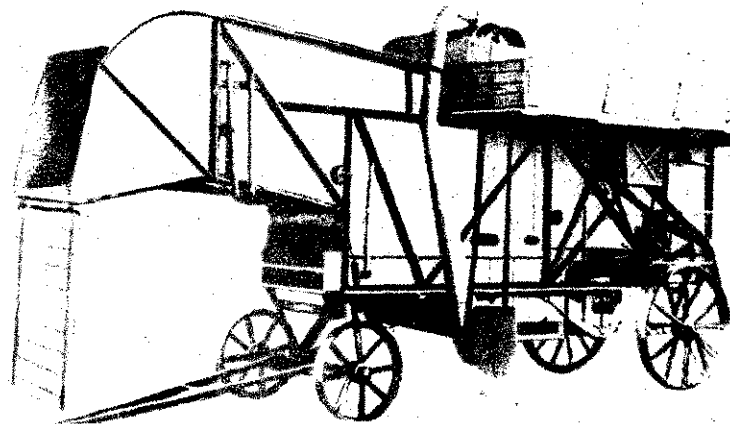
„HF“ herefejtő készülék
