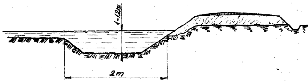
Tó mélyítés
