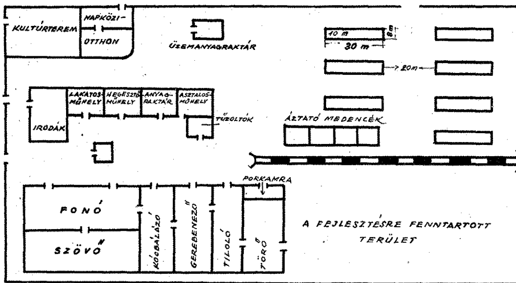
A feldolgozó részlegek elhelyezése a csarnokban
