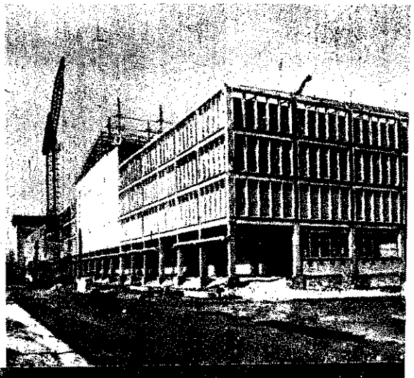
Háromezer vagonos tranzit raktár épül a Csepeli Szabványos Kikötőben. A 250 m hosszú többszintes létesítményt helyi vasbeton előgyártással építik és a kitűzött határidőre átrendeltetésének
