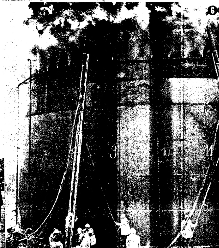
5—6. A tűzoltási kísérlet 3. napján az 1500 l/p-es teljesítményű középnyomású habsugárcsővel ellátott ügynevezett terelő habszóccokkal történt az oltás
