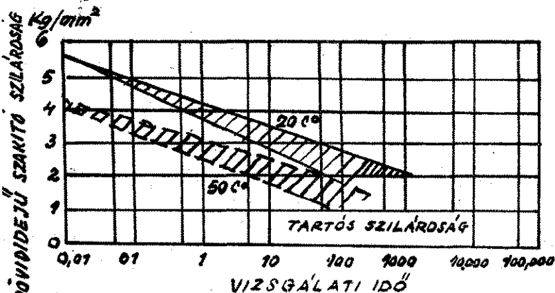
A szilárdsági értékek függése az igénybevétel időtartamától
