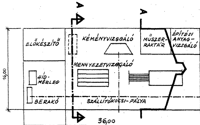
Tűzállósági minősítő laboratórium épülete
