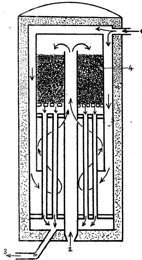
Konverter a szénmonoxid előállításához: 1. Vízgőz beáramlása — 2. Szénmonoxid beáramlása — 3. A hidrogén és a széndioxid bevezetése — 4. Krómvas-katalizátor
