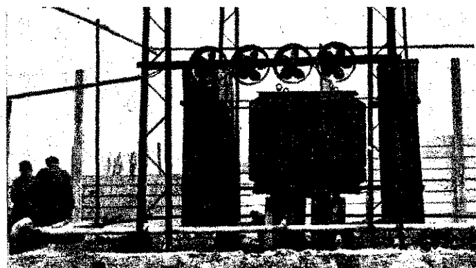
Kísérleti transzformátor 8-8 vízköd-rózsával ellátott csövezetékrendszerrel
