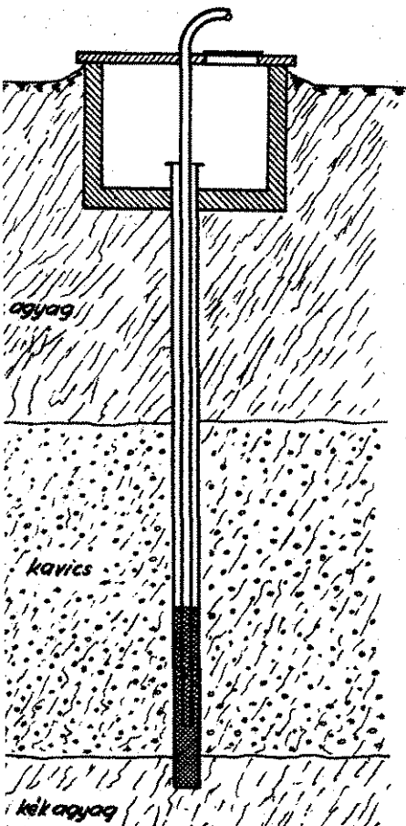
Csőkút
