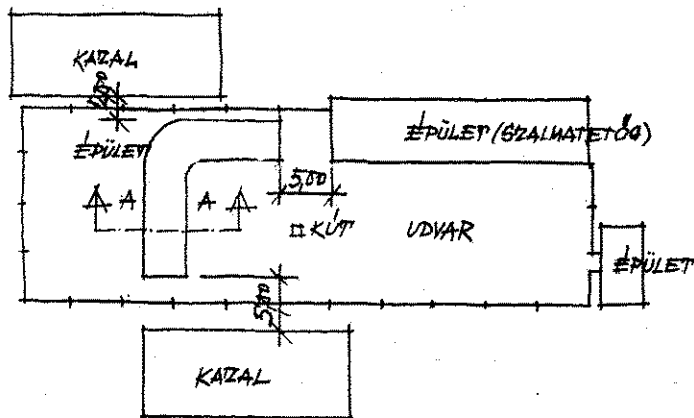
TŰZRENDESZETI SZEMPONTBÓL HELYTELENŰL TELEPÍTETT 900 FÉRŐHELYES HODÁLY TELEP
