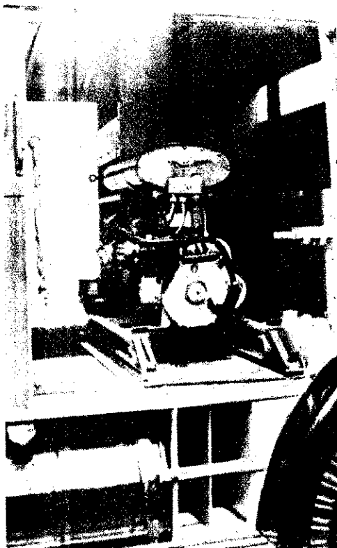
800 l/p-es kismotorfecskendő a K 300-as gépjárműn rögzítve, üzemkész állapotban, közvetlen szivatómélő csatlakozással a víztartályra
