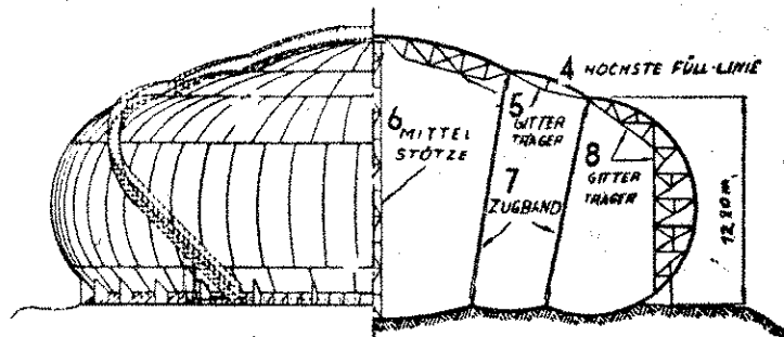
9 ANSICHT 10 SCHNITT
