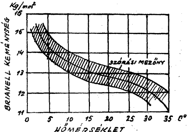
A kemény PVC felületi keménységének függése a hőmérséklettől
