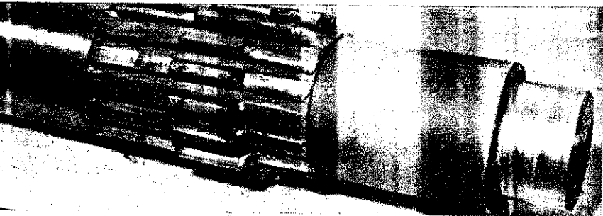
Ez a tengely a helytelen, erőszakolt sebességváltás miatt tört össze
