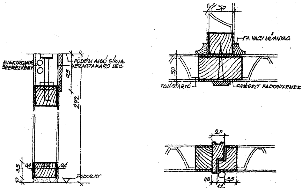
A préselt farostlemezes válaszfalak csomópontjai
