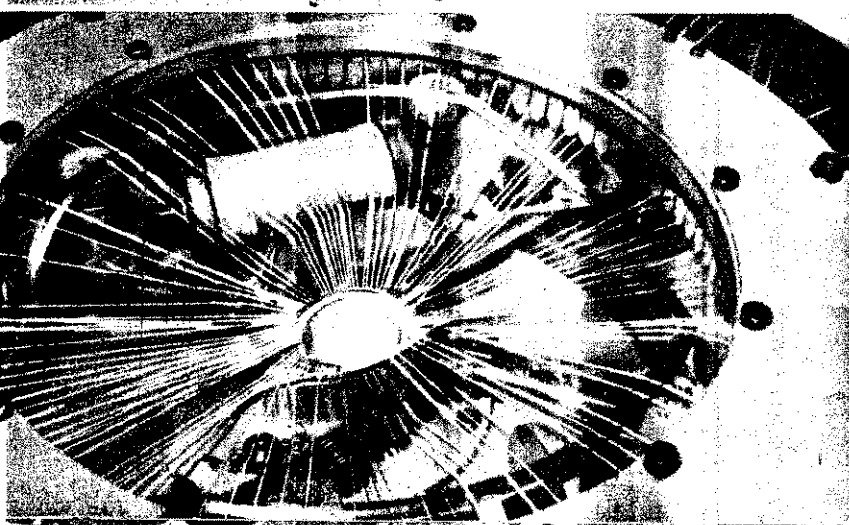
A szövőgép vetélőberendezése
