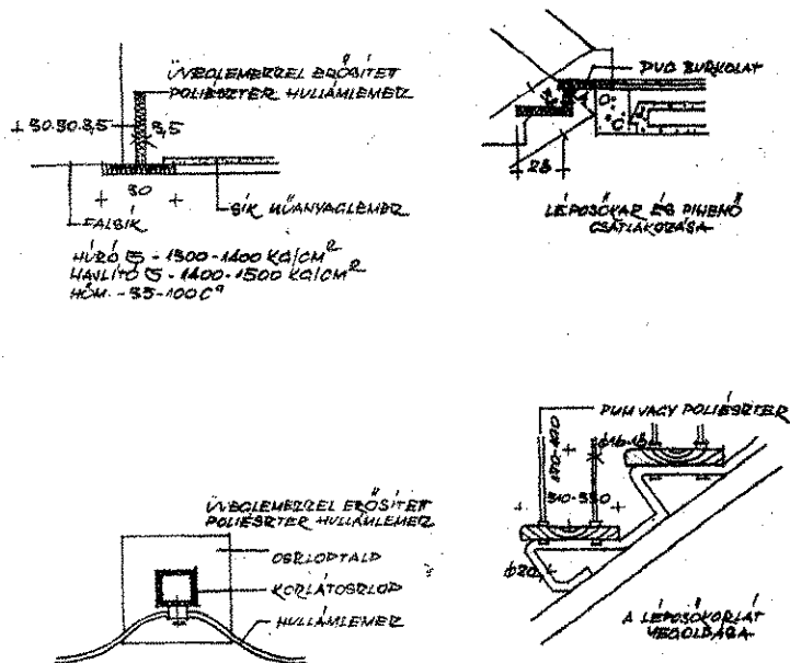
A műanyag hullámlemez alkalmazási köre
