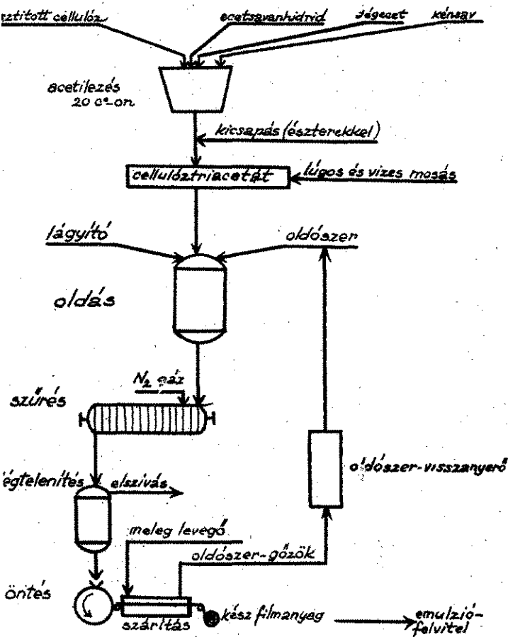
A biztonsági film gyártásának folyamata
