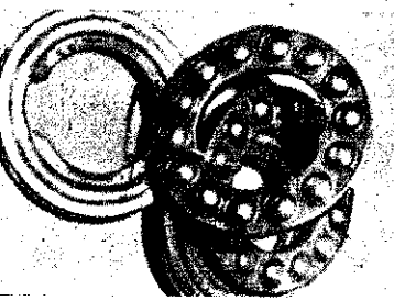
A megfelelő zsírozás elmulasztása következtében tönkrement a lánccsapágy és a szivattyútengely
