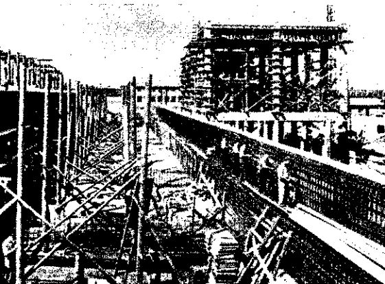
500 millió forintos beruházással új műanyaggyár épül Berentén. Az új gyár évente 6000 tonna PVC-port állít majd elő. Képfünkön: folyik a szőlő betonmedencék vasszerelése.
