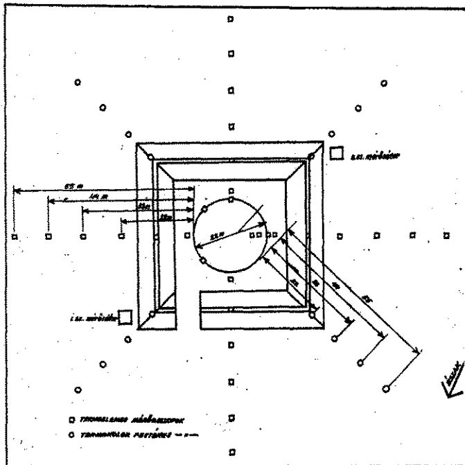
A hőmérsékleti viszonyok mérése szolgáló termoelem illetve termokolor festékek elhelyezésére szolgáló oszlop elrendezése a kísérleti tartály körül
