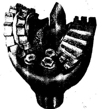
Kombinált szárnyas- és görgősfűró
