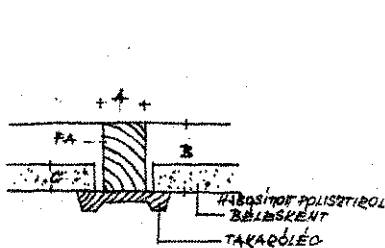
A polisztirol táblák felerősítésének módjai
