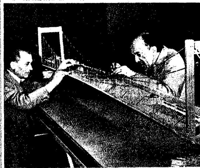
Az UVATERV modellezői elkészítették az ország első kábelhidja, az Erzsébet-híd makettjét. A makettet Vizberger Antal és Zágonyi Dezső készítették
