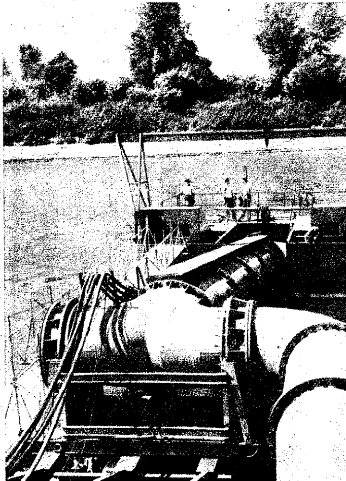
Tiszabón üzembe helyezték az ország legnagyobb teljesítményű vízvezeték-művét. Az új vízi mű a tiszavidéki állami gazdaságok és termelőszövetkezetek öntözéséhez szolgáltatja a vizet.
