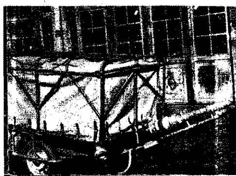
Két kép a Kísérleti Alosztály dolgozói által szerkesztett új csövázás és ponyvakáddal ellátott targoncáról
