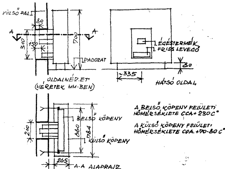
A berendezés elhelyezése külső falsíkon
