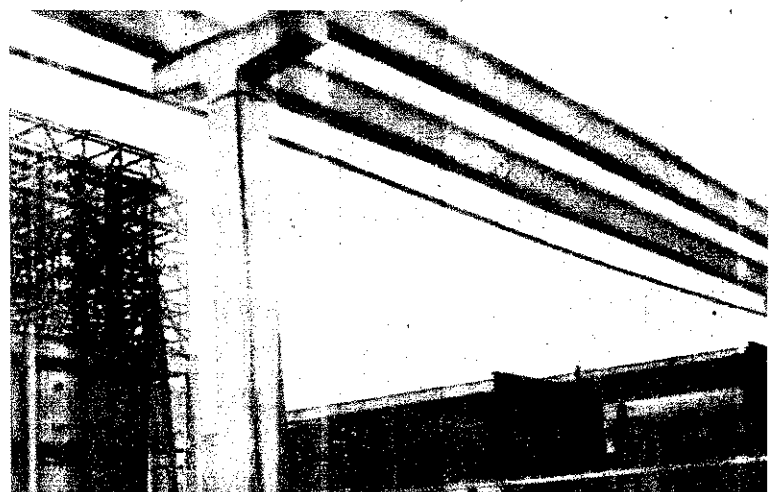
A tűz- és robbanás-veszélyes csarnokokat nagy ablakfelületekkel kellett ellátni
