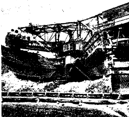
tek a hernyótalpakon mozgó hatalmas marótársas kotrógépnak az összehajlására hat hónapra volt szükség. A 5000 köbméter meddőt mozgat meg
