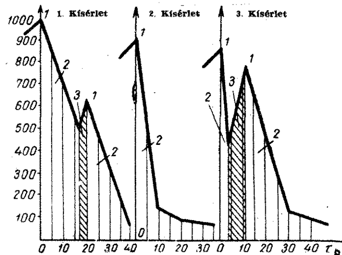
Ábrázolat a hab adagolásának hatására bekövetkezett hőmérséklet csökkenéséről. (A mérés a fűdésmeknél végezték.) 1: a habadagolás kezdetének időpontja, 2: a hab adagolásának ideje, 3: a generátor üzemzárásának időpontja. A legmagasabb hőmérsékletet a táblázat
