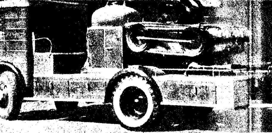
A katowiczi üzemi tűzoltóság tagjainak saját szerkesztésű porral oltó gépjárműfecskeendője
