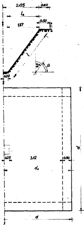
Medencebélés felületének számítása
