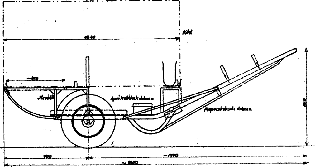
A HK-targonca oldalnézeti rajza
