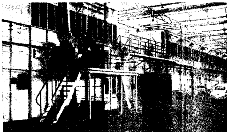
SFH-TIKKO szénssavval oltó berendezés a Volkswagen-Werk hannoveri üzemében. A szárítófülkék hátsó oldalán az oltóberendezés elosztó csővezetéke
