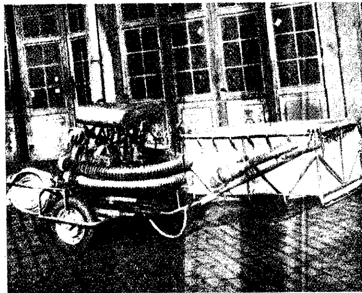
HK típusú targonca vízgyűjtőkáddal
