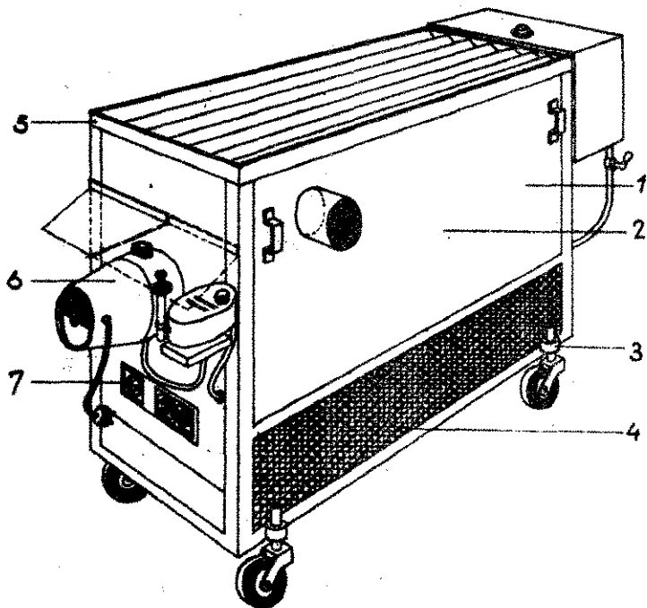
Az OT-30 típusú léghevítő fő részei: 1. léghevítő szekrény, 2. hőcserélő, 3. szállító kocsi, 4. ventilátor és elektromos szerelvény, 5. cserélhető kiftívó rács; 6. olajfűtő adagolóval és mágnesszeleppel, 7. elektromos szerelvény. A készülék üzemanyaga TH5/20 jelű tüzelőolaj, illetve téli gázolaj
