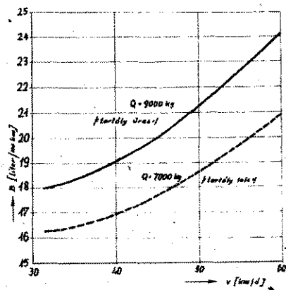
IKARUS-526 tűzoltó gépkocsi üzemanyag-fogyasztási diagramja a sebességfüggvényében.
