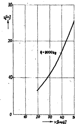
Fékút nagysága különböző sebességekről lassítva üzemi fékkel. IKARUS-526
