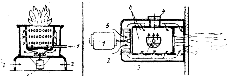
3—4. ábra: Függőleges lángrú elpárologtató égő. 1. olaj, 2. levegő, 3. ventilátor — Vízszintes lángrú elpárologtató égő: 1. motor, 2. ventilátor, 3. elpárologtató tálcá, 4. gyújtónyílás, 5. levegőbevezetés, 6. primer levegő, 7. szekunder levegő
