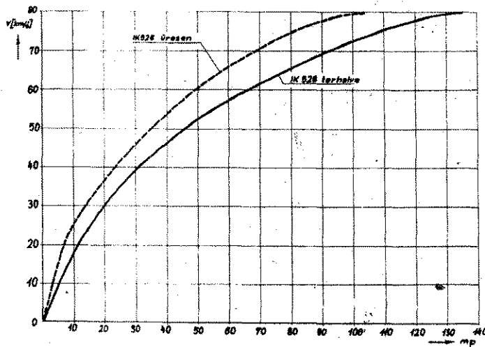
IKARUS-526 típusú tűzoltó gépkocsi gyorsulási diagramja.
