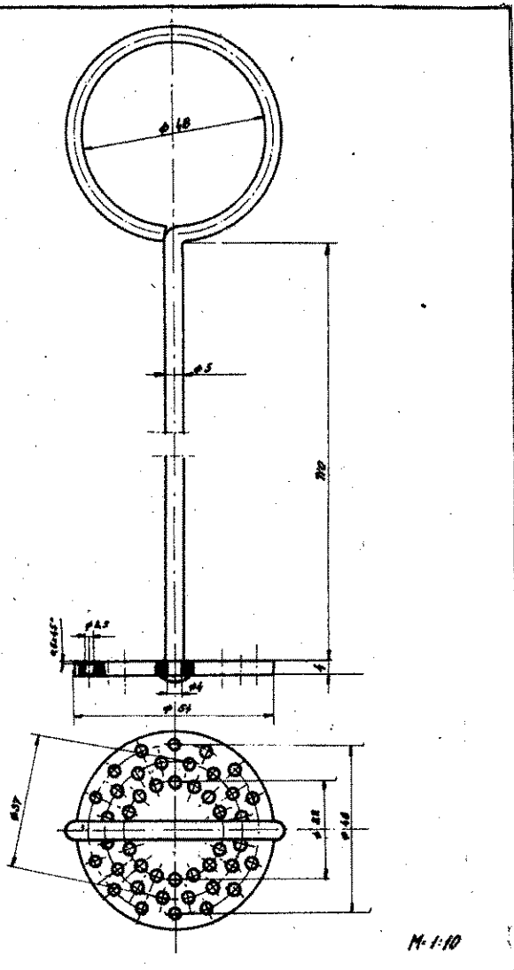
A habverő (anyaga alumínium) méretarányos rajza
