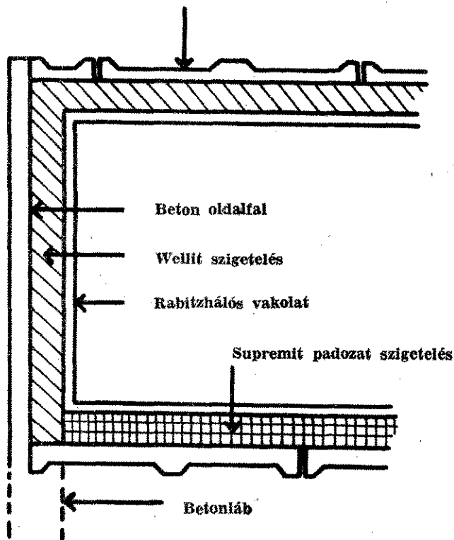
A hőszigetelt helyiségek keresztmetszete. A rajz jól szemlélteti a hűtőháznál alkalmazott építő-, illetve szigetelőanyagok beépítési módját
