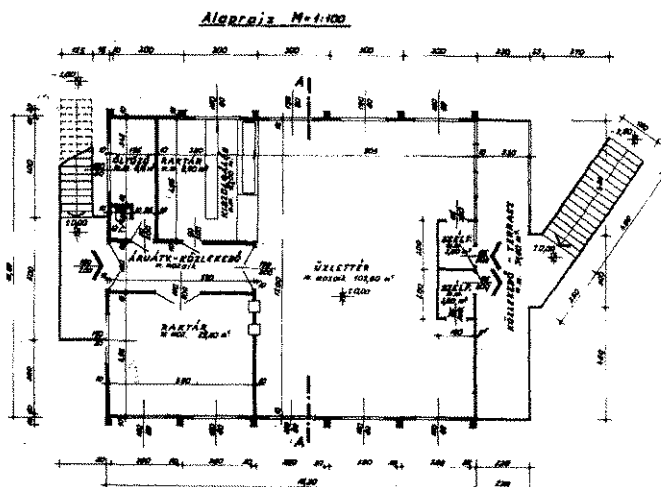
Éghető anyagú szendvicspanelből épített élelmiszer-áruház alaprajza
