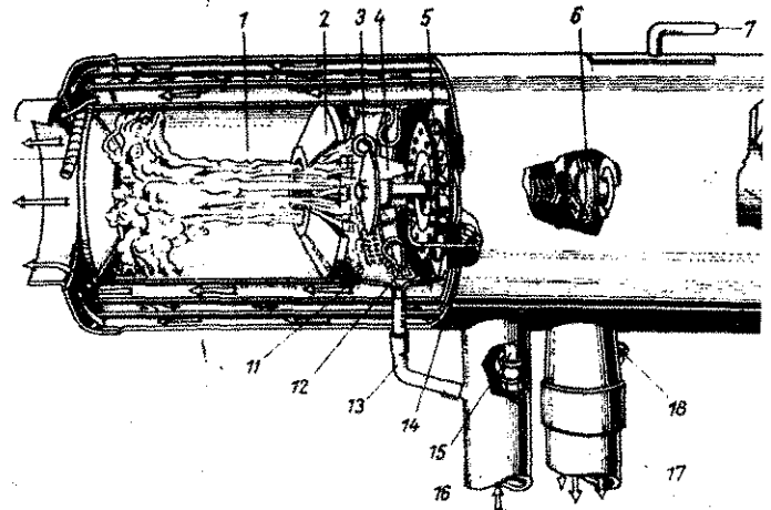
6. ábra: IKALOR légfűtő berendezés. 1. tüzelőtér, 2. lángszűkítő, 3. izzó-gyertya, 4. szórókúp, 5. égéslevegő-járókerék, 6. tengelyk 7. tengelykapcsoló-kézikar, 8. ventilátor, 9. villanymotor, 10. tűh dőst gátló bimetallickapcsoló, 11. égőtér, 12. olajnyomócső, 13. olaj folyócső, 14. olajszivattyú, 15. olajvezeték, 16. égéshez szükséges szívócső, 17. kipufogó, 18. égést ellenőrző bimetallic kapcsoló
