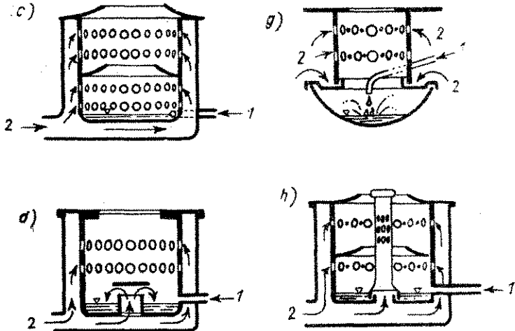
1—2. ábra: c) tálcás égő két torlógyűrűvel, d) tálcás égő egy torlógyűrűvel, 1. olajbevezetés, 2. levegőbevezetés — g) zárt, csepegtető rendszerű tálcás égő, h) tálcás égő két torlógyűrűvel, zárt részben központi levegőbevezetéssel, 1. olajbevezetés, 2. levegőbevezetés
