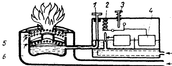
5. ábra: Elpárologtató rendszerű égő két üszös adagolóval. 1. kézi s lyező szelep, 2. rugó, 3. üsző, 4. biztonsági üsző, 5. szekunder levegő primer levegő, 7. olajvezetés, 8. levegőbevezetés
