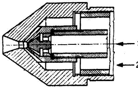
13. ábra. Perédi-féle égőfej
