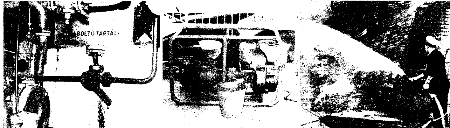
A „Hunyadi” tűzoltófelszerelése: a haboltó tartály, a 400-as hordozható szivattyú és a 200/2-es habugárcső
