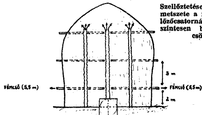
Szellőztetéses kazal oldalnézetben a függőleges szellőzőcsatornákkal és a fémcsövek végeivel
