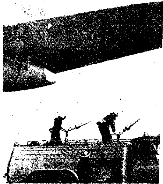
„Tatra 138” típusú, 3200-as tartályos gépjárműfecskendőt állított szolgálatba az NDK tűzoltósága a Berlin-Schönefeld-i repülőtéren. A gépjármű 6000 liter vizet és 600 liter habképző anyagot szállít, 180 LE teljesítményű motorja 3200-as szivattyút hajt. A speciálszernek 2 db hab-, illetve vízágyúja is van
