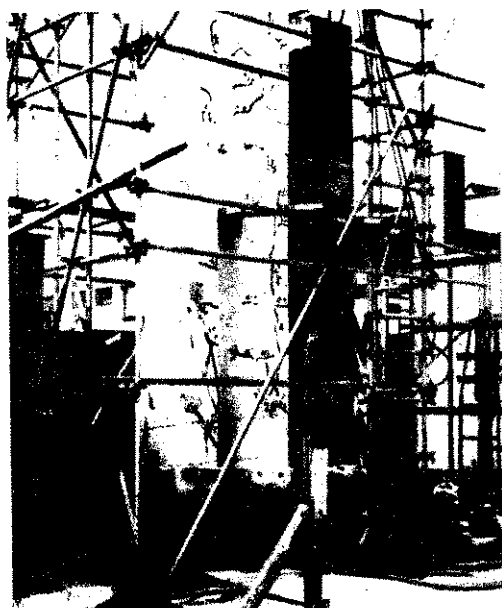
Téglazúzalék-adalékos kémények repedése képe, az I. jelű (bal oldali) és a II. jelű (jobb oldali) — tűzpróba után
