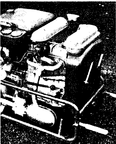
A közelmúltban kiadott, Skoda motorral ellátott legújabb 1200 l/p-es kis-motorfecskendő
