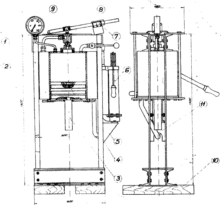
1: vázszerkezet 2: olajtartály; 3: dugattyúrúd; 4: háromrészes dugattyú; 5: munkahenger; 6: dugattyús szivattyú; 7: mérlegkar, súly, rögzítő; 8: súlyszelep; 9: feszmérő; 10: vázszerkezet-talp; 11: dug. szív. bak.
