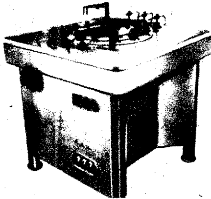
Az FGYF—0764 típusú, 12 fejes dióda-bevezető-gyöngyözőgép
