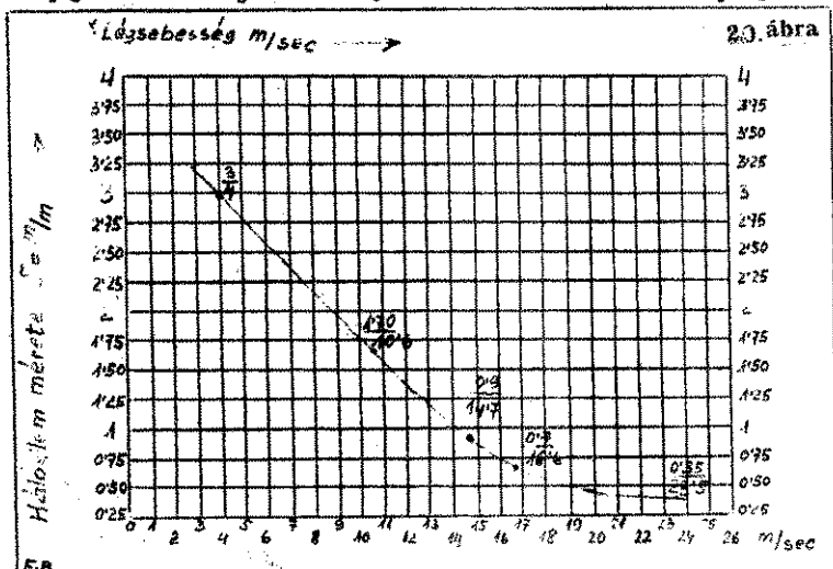
Habfejlesztés a levegő sebesség és a szita szem méretének függvényében.
