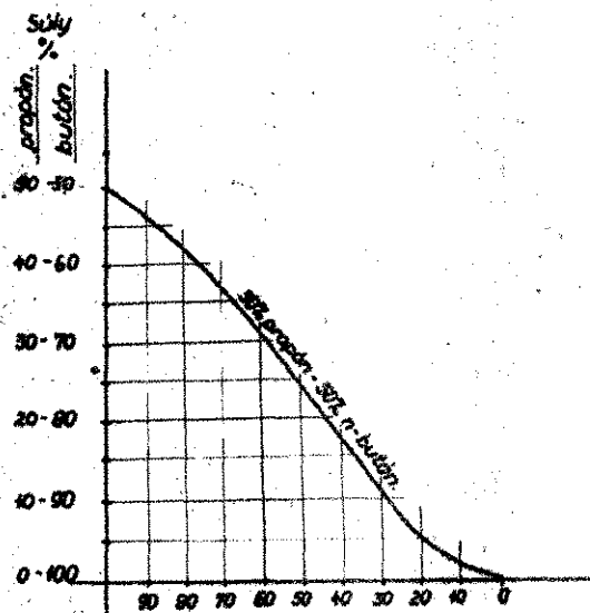
Maradék palack-töltet a teljes töltet %-ában.
