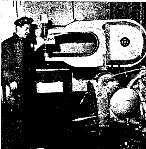
A Polgár – Konkoly – Borbás-féle villamos ponthegesztő készülék „nyugalomban” és munka közben
