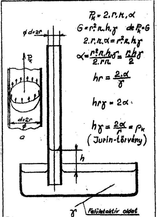
A kapilláris erő mérése
