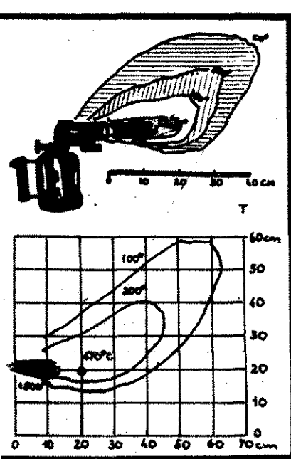
6. ábra: 1/2 és 1 literes benzín- lámpa lángjának hő- mérséklet-eloszlása
