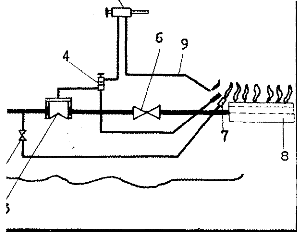
Ligeti-típusú kazán égésbiztosító és hőmérséklet-szabályozó automatikája
