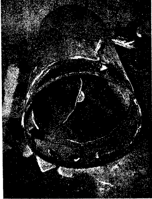
A kazán vízköpenyének felhasadása
