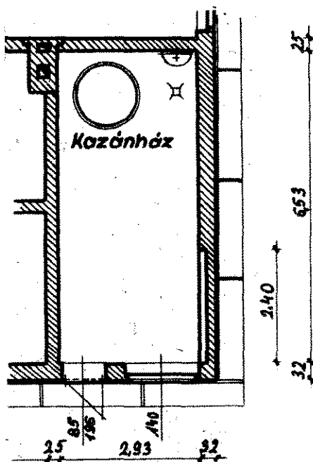
A kárhely alaprajza
