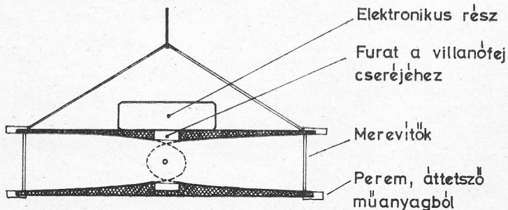
7. ábra. A világítóegység forgási-parabola tükrökkel A villanófej a közös fókuszba kerül
