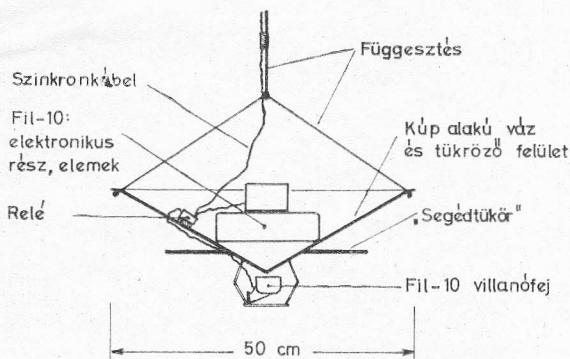
2. ábra. A szelvényvilágító metszete
