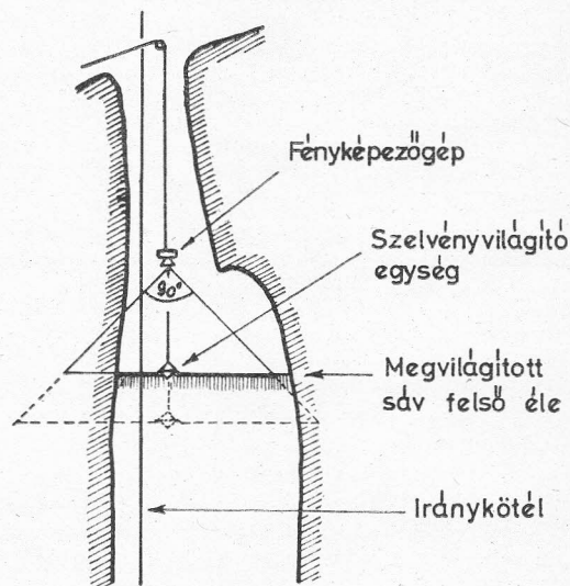
3. ábra. A mérés elve. A megvilágítási távolság és a látószög összefüggése
