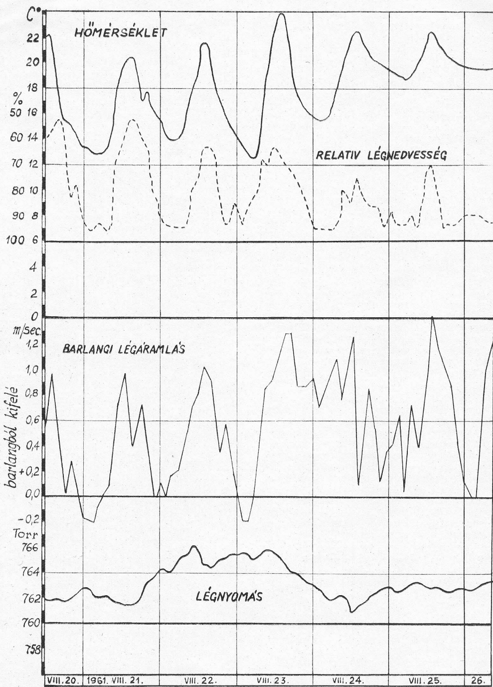
4. ábra. A barlangi légáramlás és az időjárási elemek alakulása közötti összefüggés grafikus szemléltetése (nyári mérésorozat)
