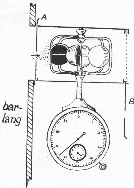
2. ábra. A barlangi levegő ki-beáramlásának mérése szolgáló egyszerű szerkezet kézi kanalas anemométer beépítésével a barlang bejárati ajtaján
