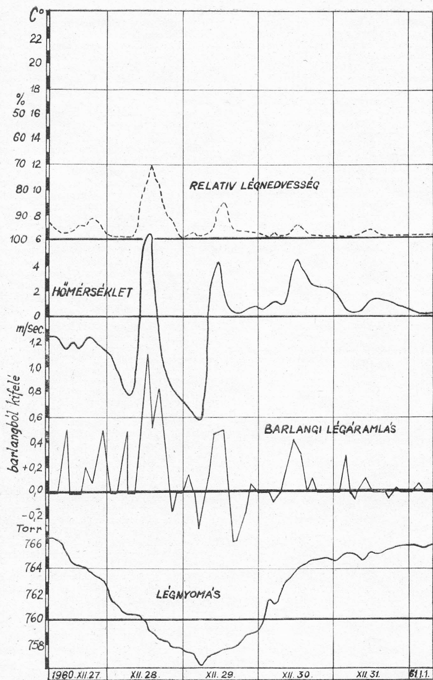
5. ábra. A barlangi légáramlás és az időjárási elemek alakulása közötti összefüggés grafikus szemléltetése (téli — mérőszorozat)
