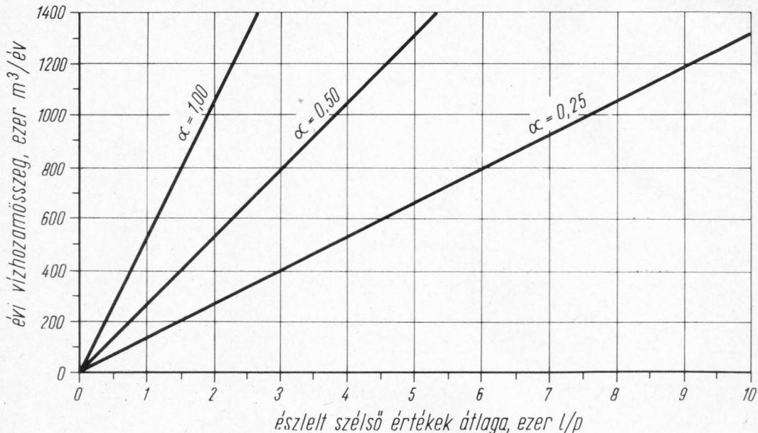
1. ábra. Segédlet az évi vízhozamösszegek számításához
