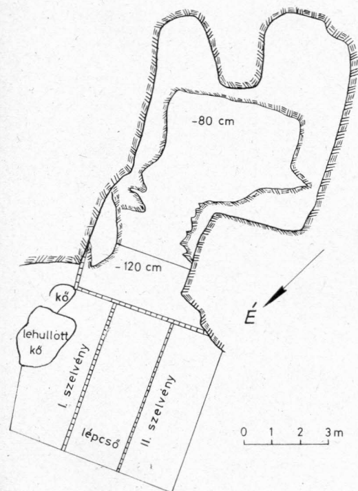
A Diósgyőr—Tapolca-barlang vázlatos alaprajza
