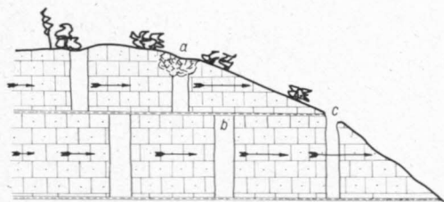
8. ábra. A barlangok kialakulásának modellje
