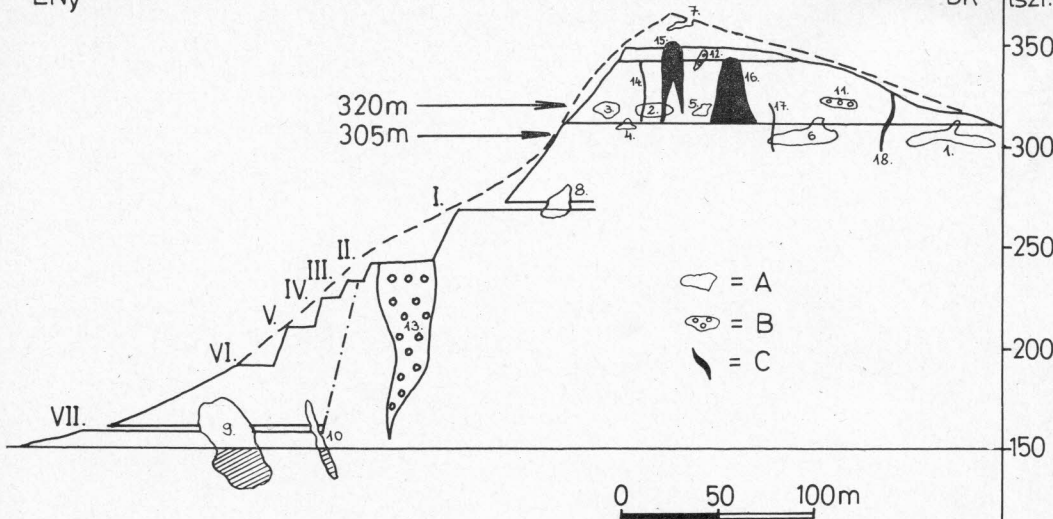
1. ábra. Az Esztramos-hegy sématiszus metszete (Pantó G. után Kiegészítve). A = barlangok, B = fosszilis barlangok, C = hasadékok, 1 = Esztramosi-barlang, 2 = Felső 2. számú barlang, 3 = Felső 3. számú barlang, 4 = Felső 4. számú barlang, 5 = Felső 5. számú barlang, 6 = Felső 6. számú barlang, 7 = Csúcs alatti-barlang, 8 = 1-es szint barlangja, 9 = Rákóczi 1. számú barlang, 10 = Rákóczi 2. számú barlang, 11 = 2-es gerinces lelőhely fosszilis barlangja, 12 = 3-as gerinces lelőhely fosszilis barlangja, 13 = fosszilis barlang 14 = 14-es gerinces lelőhely, 15 = 1-es gerinces lelőhely, 16 = középső pleisztocén korú hasadék, 17 = 8-as gerinces lelőhely hasadéka, 18 = 7-es gerinces lelőhely
