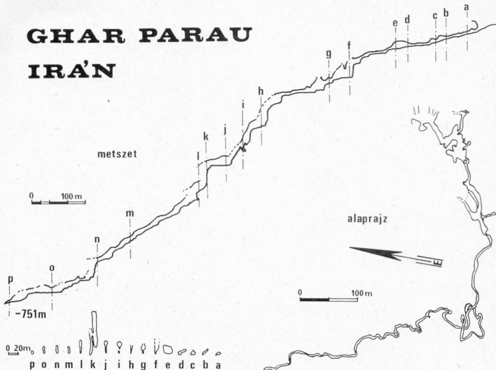
A Ghar Parau-barlang térképe
