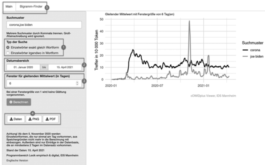
Abb. 1: Startseite des cOWIDplus Viewer (mit hervorgehobenen Bereichen, auf die wir im Text Bezug nehmen)
