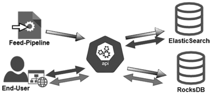
Abb. 2: OWIDplusLIVE verteiltes Konzept
