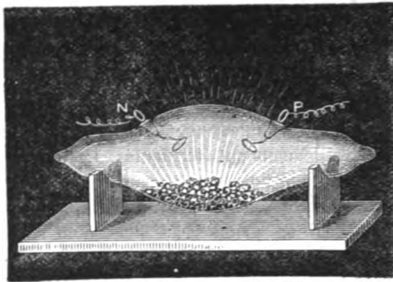
MATIÈRE RADIANTE. — Expérience de Crookes.
