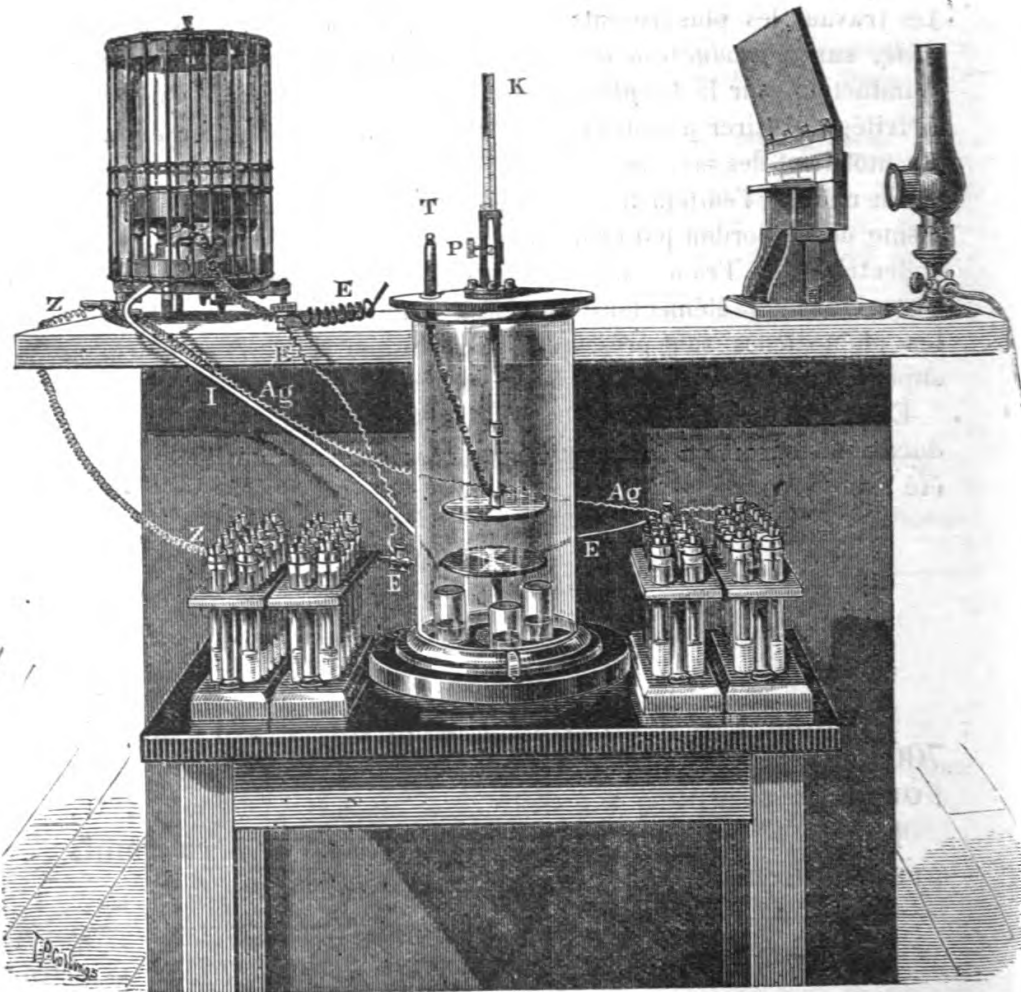
DÉCHARGES DANS LE VIDE. — Électromètre symétrique de Warren De la Rue.
