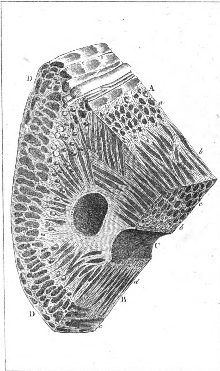
Coupes de la Trompe de l'Éléphant .
