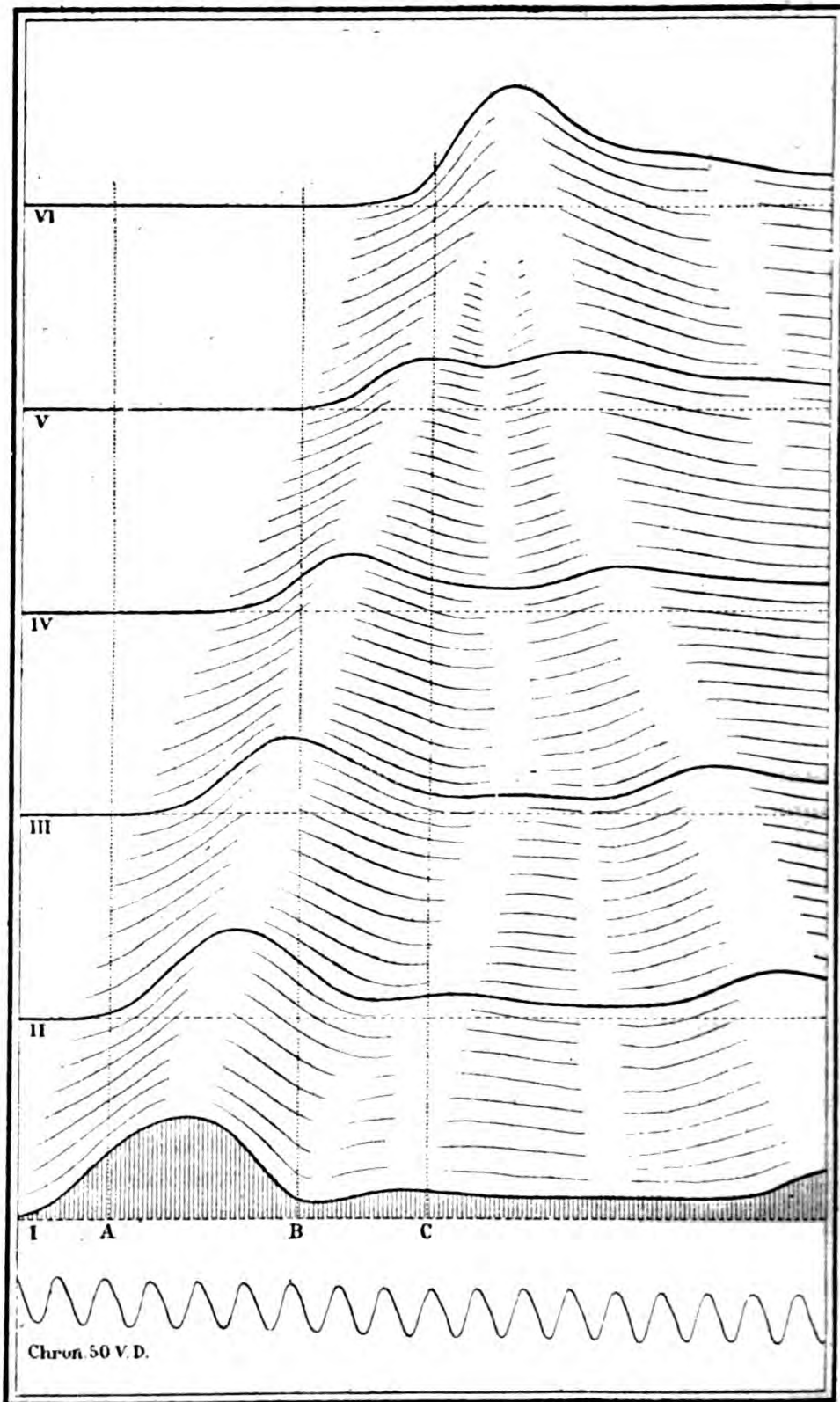
Fig. 63. — Représentation stéréoscopique du trajet de l'onde.
