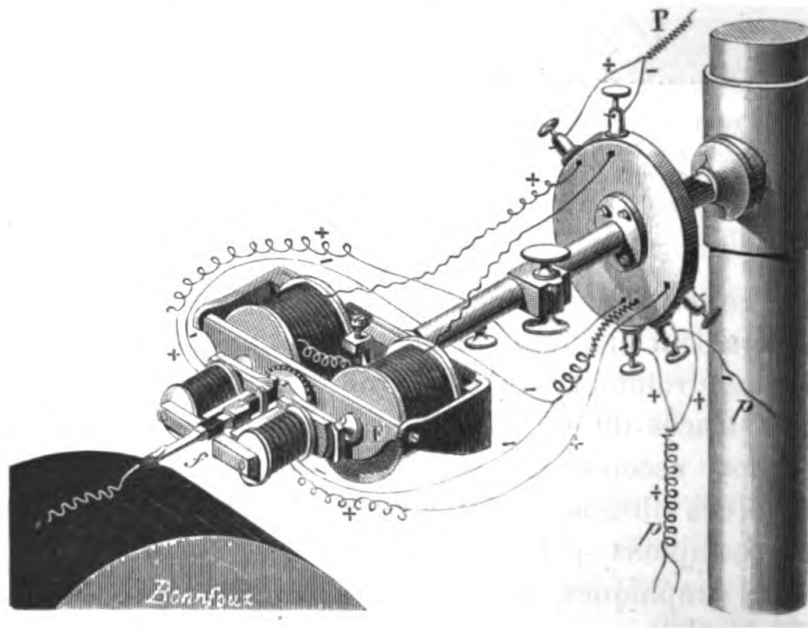
FIG. 115 Chronographe inscrivant cent vibrations par seconde.
