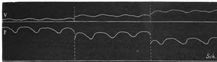
Fig. 158. — Ajutage d'écoulements de plus en plus large; la vitesse et la pression varient en sens inverse.
