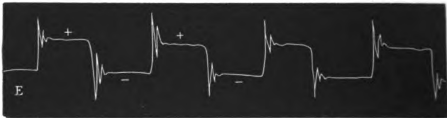
Fig. 56. — Ondes produites par les oscillations d'une colonne d'eau dans un tube, inscrites à l'aide d'un sphygmographe.
