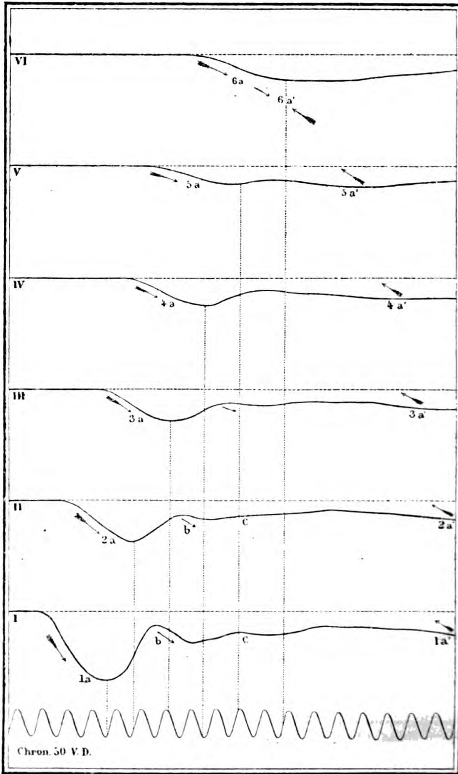
Fig 62. — Onde negative dans un tube fermé.
