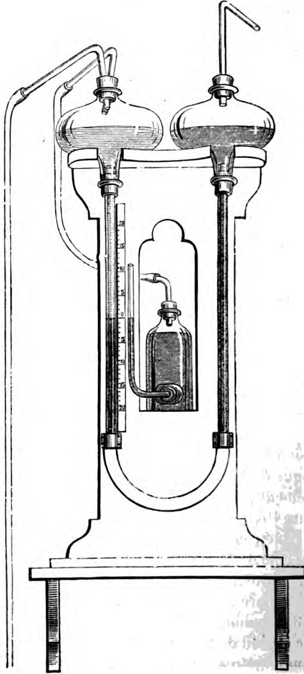
Fig. 109. — Manomètre à deux liquides.
