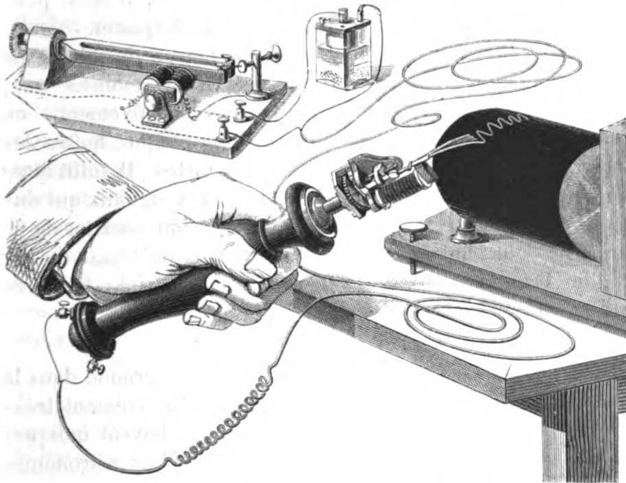
Fig. 73. — Chronographe tenu a la main et donnant continuellement 100 vibrations doubles par seconde.
