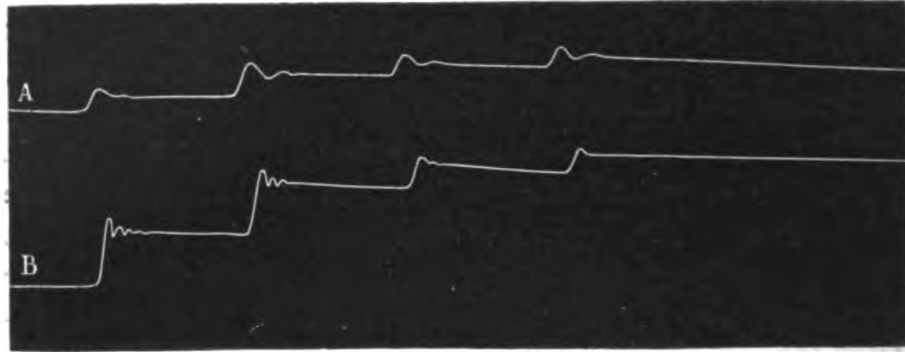
Fig. 66. — A et B, pulsations recueillies dans deux tubes branches sur un même réservoir comme les artères sur l'aorte. — A, tube long. — B, tube court.
