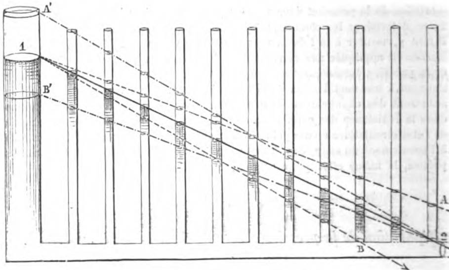
Fig. 143. — Piézomètres et variations de leurs niveaux suivant les changements dans l'afflux ou l'écoulement du liquide.
