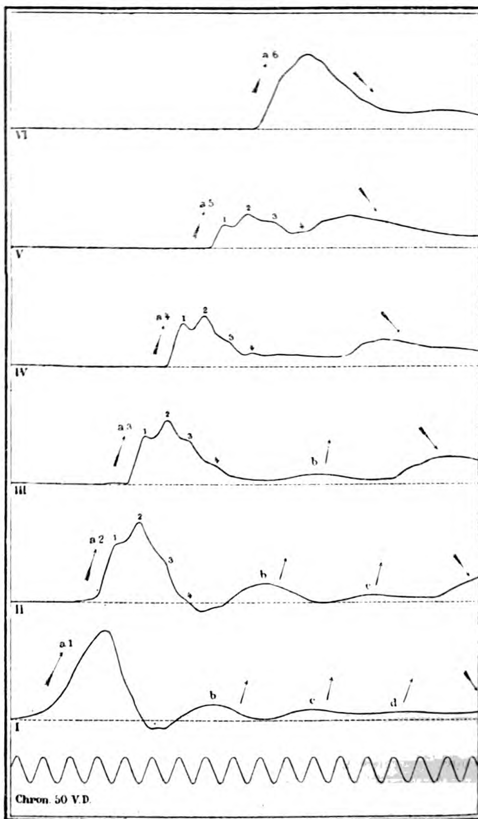
Fig. 64. — Ondes de second ordre ou harmoniques, dans un tube fermé.
