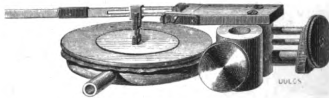
Fig. 17. Tambour à levier perfectionné
