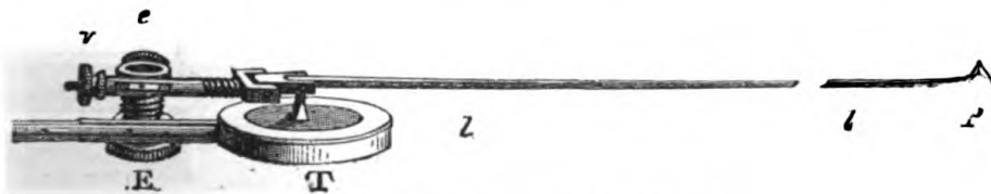
Fig. 10. — Tambour à levier enregistreur.
