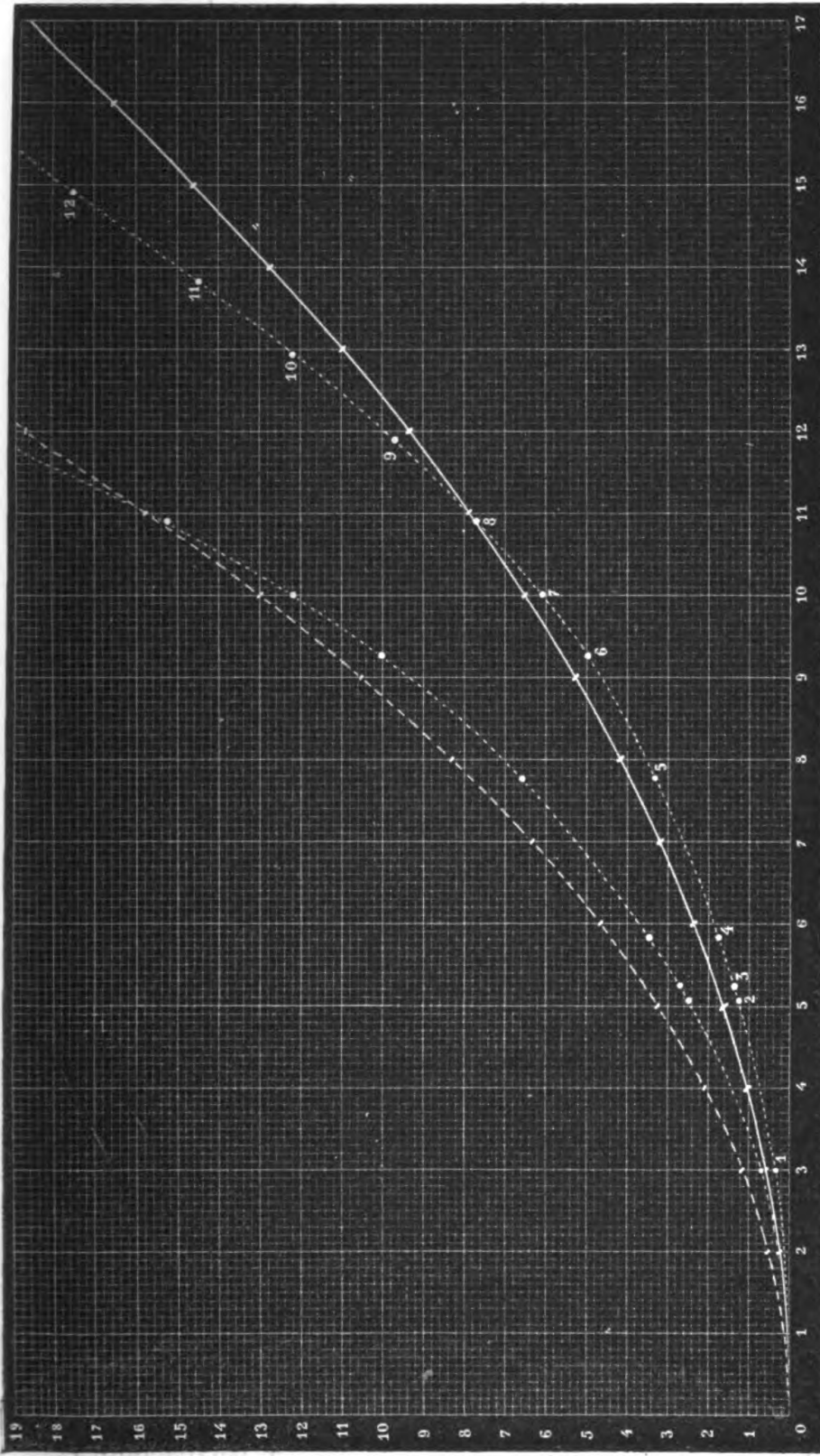
Fig. 118. — TABLEAU II. — La courbe construite par une série de points dont chacun porte un numéro d'ordre exprime l'accroissement de la pression au devant d'un plan d'un mètre de surface, pression calculée d'après l'aspiration centrifuge. — La courbe construite au-dessus de celle-ci par une série de points sans numéros d'ordre a des ordonnées doubles de la précédente; ce serait celle de la résistance de l'air d'après les expériences. — La courbe pleine exprime la pression de l'air au devant d'un plan, en admettant, pour un mètre carré de surface animé d'une vitesse d'un mètre, une pression de 65 grammes et en supposant que cette pression croisse comme le carré des vitesses. — Enfin, la courbe supérieure formée de traits serait, d'après la même hypothèse, celle de la résistance de l'air.
