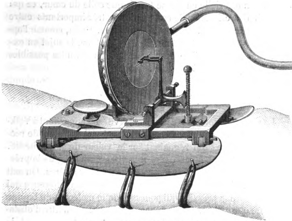
Fig. 142. — Sphygmographe à transmission.
