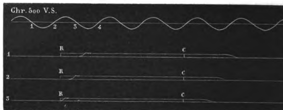
Fig. 79. — Trace supérieure chronographe de 500 vibrations simples ; les chiffres 1, 2, 3, 4, marquent les temps correspondant à \frac{1}{500} de seconde. — Ligne 1, R, instant de la rupture du courant de pile. La courbe qui, partant de la ligne inférieure, s'élève obliquement à la ligne supérieure, est le mouvement du style au moment où la désaimantation se produit. La durée du retard mesuré sur le chronographe dépasse \frac{1}{500} de seconde ; c'est le retard de désaimantation. C, clôture du courant de pile : le moment où la ligne supérieure redescend au contact de l'inférieure correspond au signal d'aimantation ; son retard est de \frac{1}{500} de seconde environ. — Ligne 2 et 3. Diminution graduelle des retards de désaimantation et d'aimantation.
