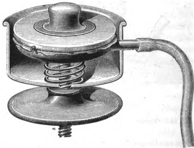
Fig. 15. — Explorateur à tambour applicable sur l'homme et sur les animaux. — En tournant la vis de réglage, on fait saillir plus ou moins le bouton de l'explorateur ce qui augmente ou diminue la sensibilité de l'instrument. (La cloche de bois a été coupée par sa moitié, pour laisser voir les pièces intérieures.)
