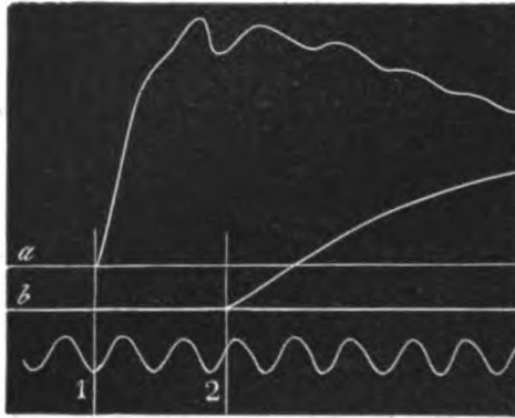
Fig. 78. — Mesure de la vitesse de transmission des signaux dans les tubes à air. Ligne a , signal 1, retard pour 1 mètre de tube. Ligne b , signal 2, retard pour 31 mètres. Différence, 2\frac{1}{3} vibrations de 250 par seconde. — Vitesse, 325 m.
