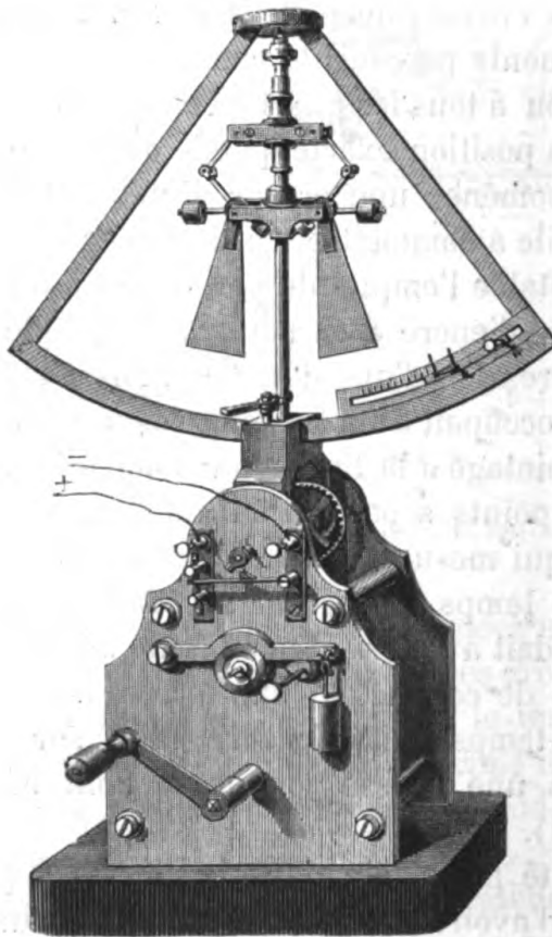
Fig. 70. — Mouvement d'horlogerie muni du régulateur Villarceau. Cet appareil est destiné à faire tourner uniformément le cylindre sur lequel on inscrit les signaux.
