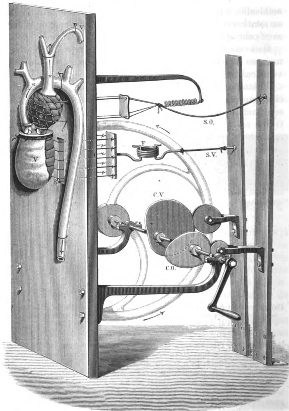
Fig 45. — Schéma de la circulation du sang.
