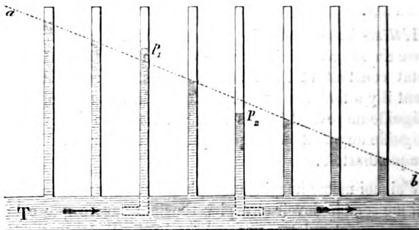
Fig. 143. — Tube T dans lequel se fait un écoulement de liquide dans le sens des flèches a, b , niveaux d'une série de piézomètres. — P_1 et P_2 , tubes de Pitot, diversement orientés; leurs niveaux diffèrent de ceux des piézomètres.
