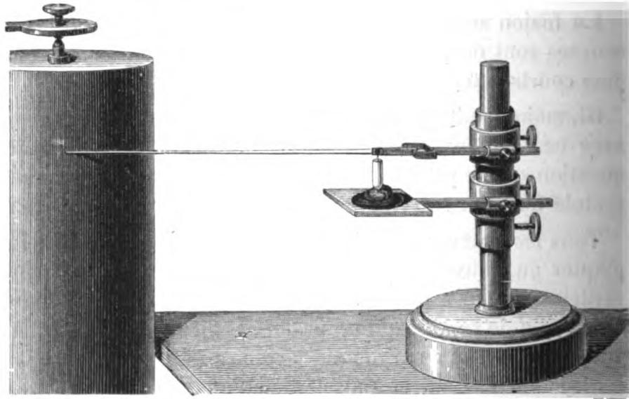
[Fig. 23. — Myographe du cœur.
