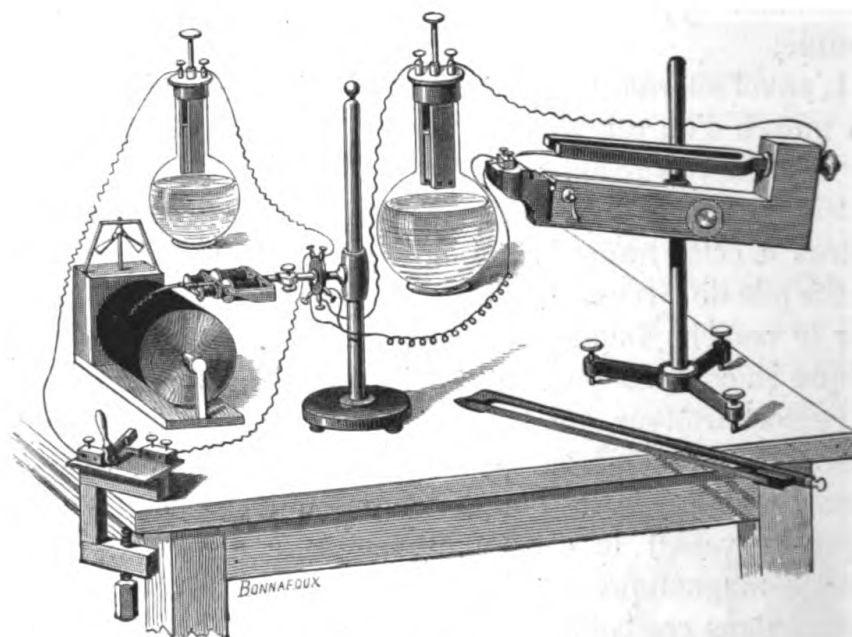
FIG. 116. — Disposition générale des appareils chronographiques.
