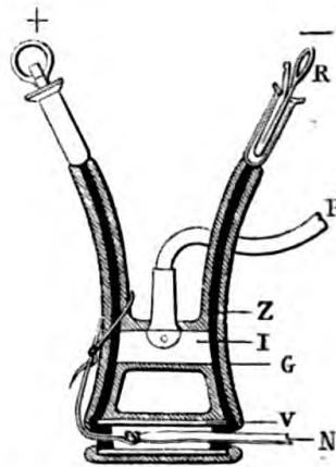
Fig. 157. Excitateur isolé. — P, tige en plomb fixée à une plaque d'ivoire ; Z, tige de zinc amalgamé formant conducteur ; V, tube de verre isolant les deux zincs ; G, gutta-percha isolant l'appareil ; N, nerf introduit dans le tube excitateur et fixé avec un fil. (Le fil doit toujours être introduit par le plus petit orifice avant la ligature du nerf : c'est par le glissement de ce fil dans l'anneau qu'on attire le nerf dans le tube).
