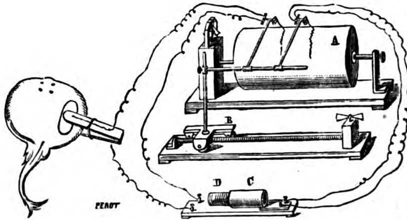
Fig. 1. — Une Torpille est saisie entre les mors d'une pince qui recueille les décharges électriques et les envoie à un signal de Deprez qui les inscrit sur un cylindre; en même temps les décharges traversent la bobine inductrice D. Un autre signal, placé sur le circuit de la bobine induite C, inscrit les courants induits par la décharge.
