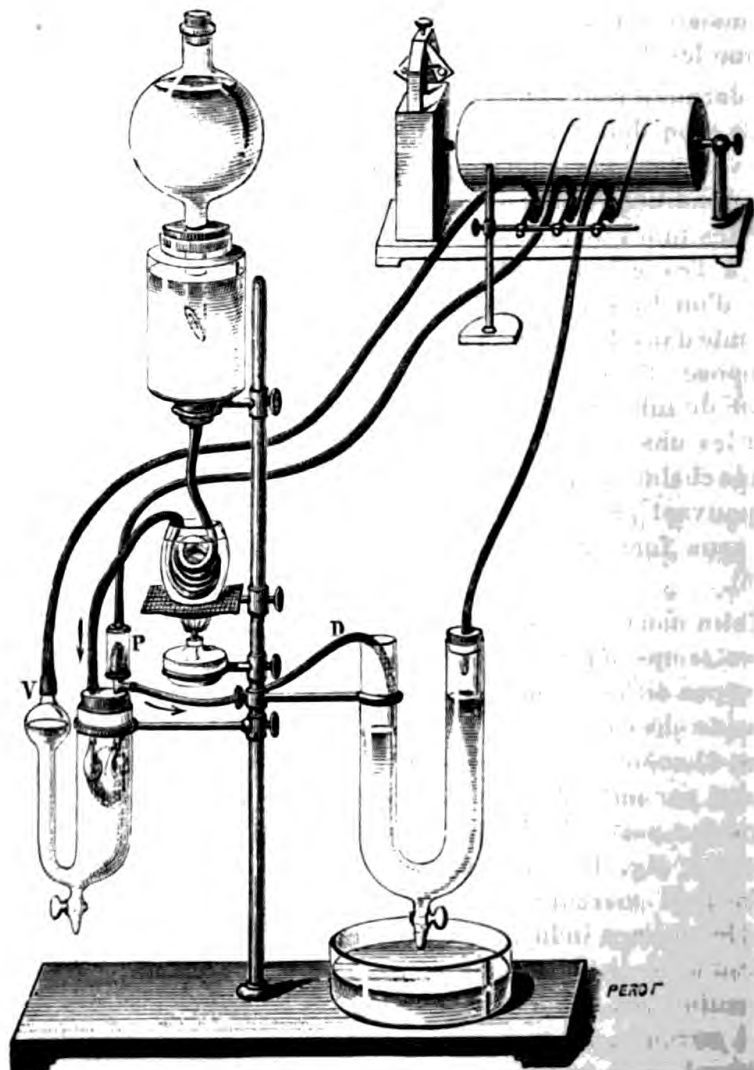
Fig. 151. Appareil à circulation artificielle pour le cœur de la tortue, permettant d'étudier les changements de volume du cœur (v), les variations de la pression artérielle (P) et les débits (D) correspondant aux systoles. — (Les hauteurs des niveaux du sang dans le tube en U où se fait l'écoulement D doivent être interverties.)
