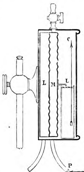
Fig. 150. — Manomètre à cadran et à transmission.
