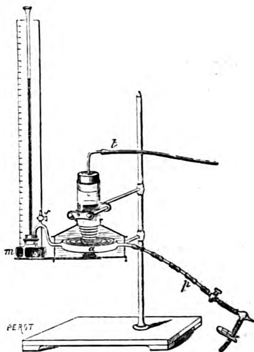
Fig. 148.— Manomètre métallique monté et prêt à fonctionner.
