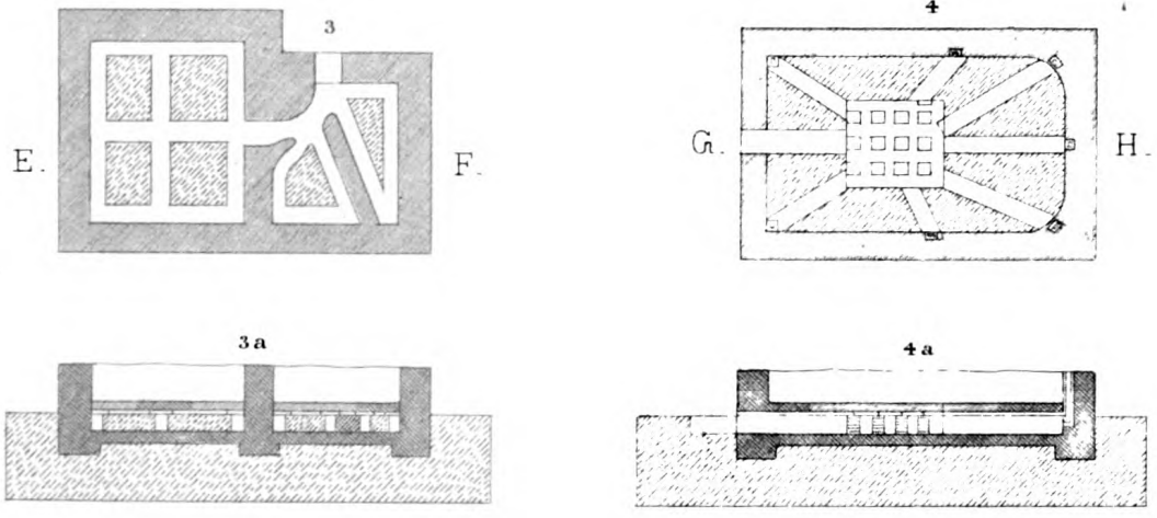
SCHNITT E-F-
