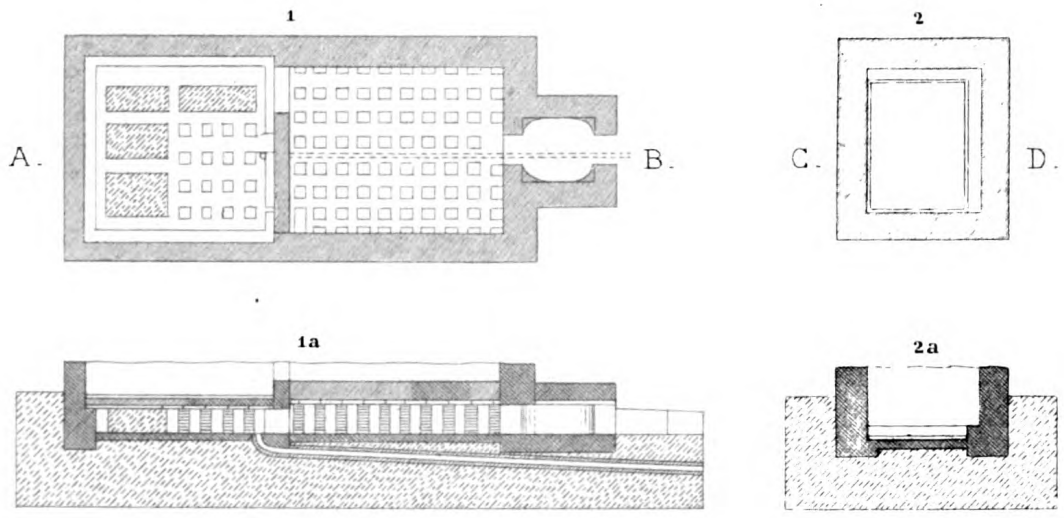
SCHNITT-A-B-
