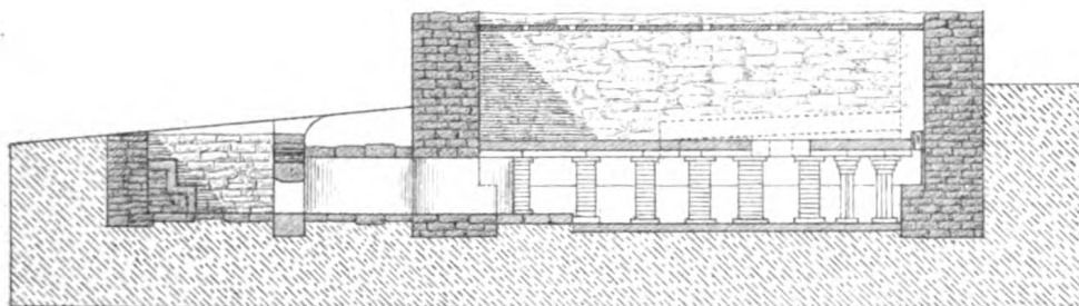
SCHNITT-A-B-
