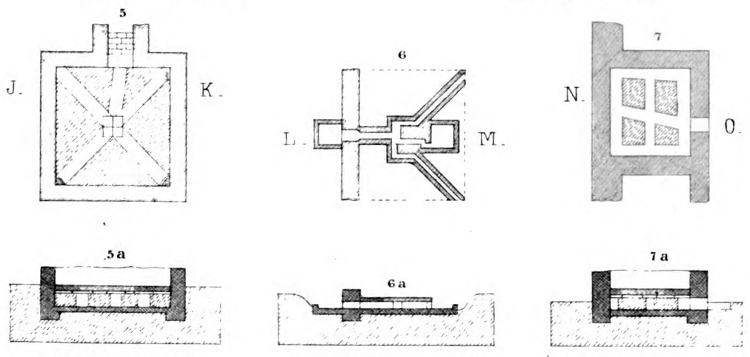
SCHNITT-L-M-
