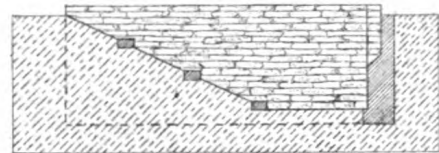
SCHNITT-J-K-
