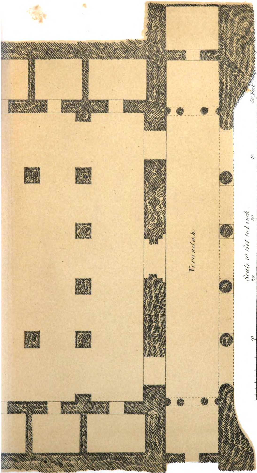
PLAN OF VIHARA CAVE N o 2 ATAJUNTA.
