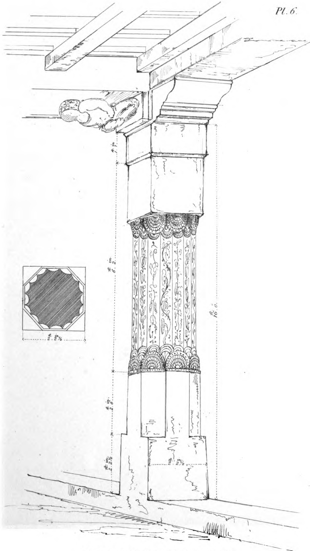
PILLAR IN CAVE N° 17. AT AJUNTA.
