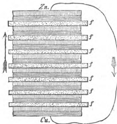
Fig. 123.—VOLTAIC PILE.
