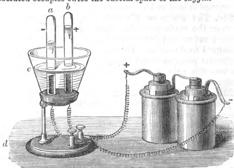
Faraday's Voltameter.
