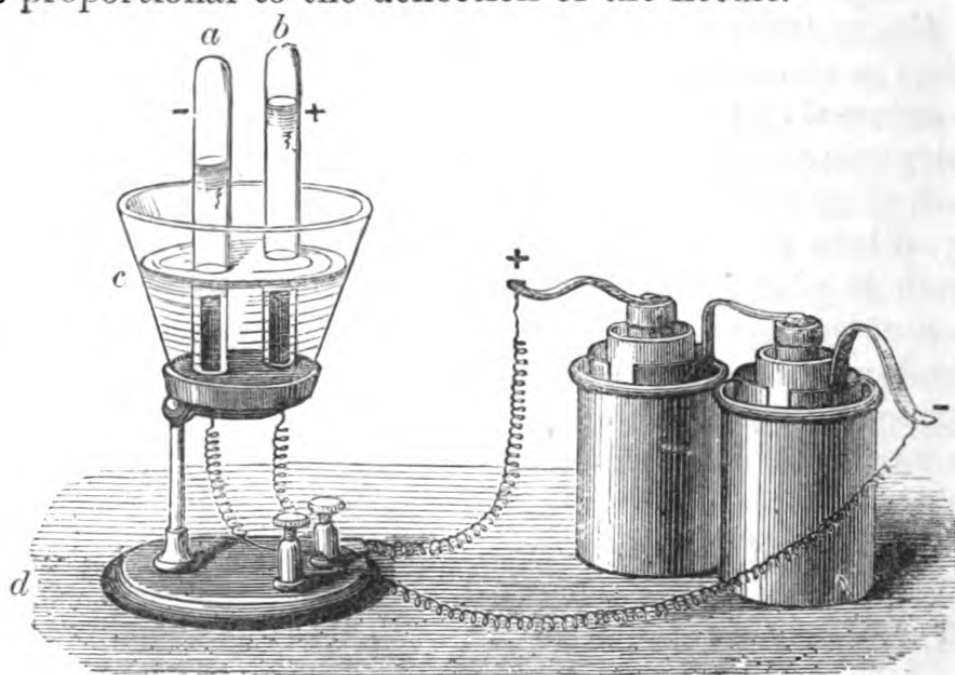
Faraday's Voltameter.
