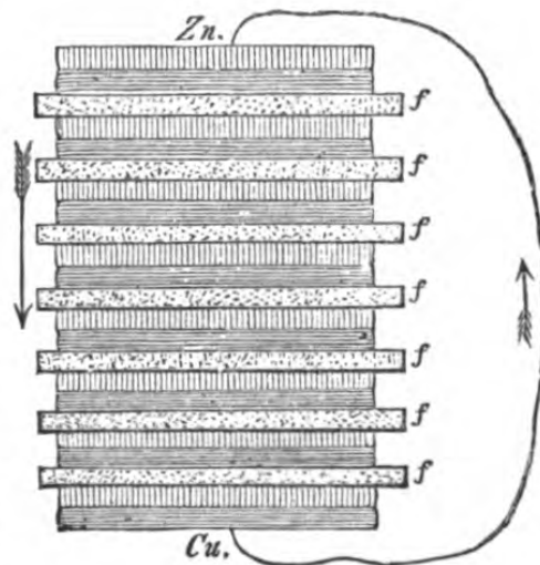
Fig. 109.—VOLTAIC PILE.
